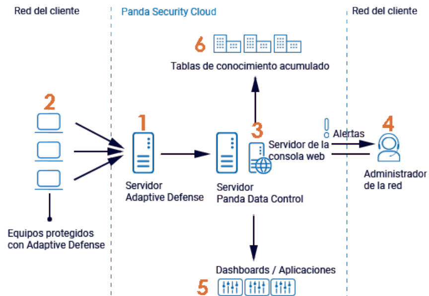
Figura 2.1: arquitectura general de Panda Data Control
